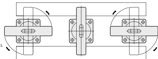
Poloha palce při upnutí materiálu
