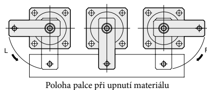
Poloha palce při upnutí materiálu
