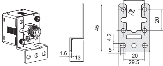
Adaptér pro montáž do panelu s ochranným krytem PA-D
