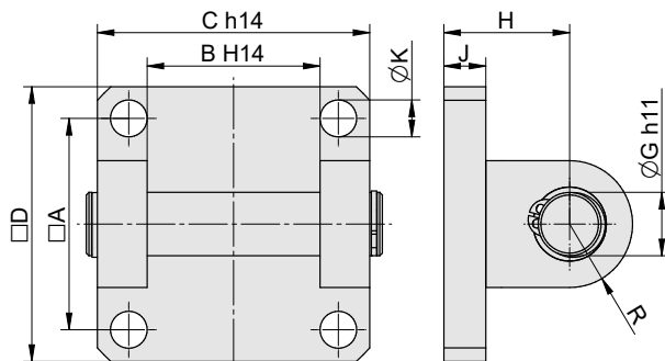
Swivel flange (page 4-19)
